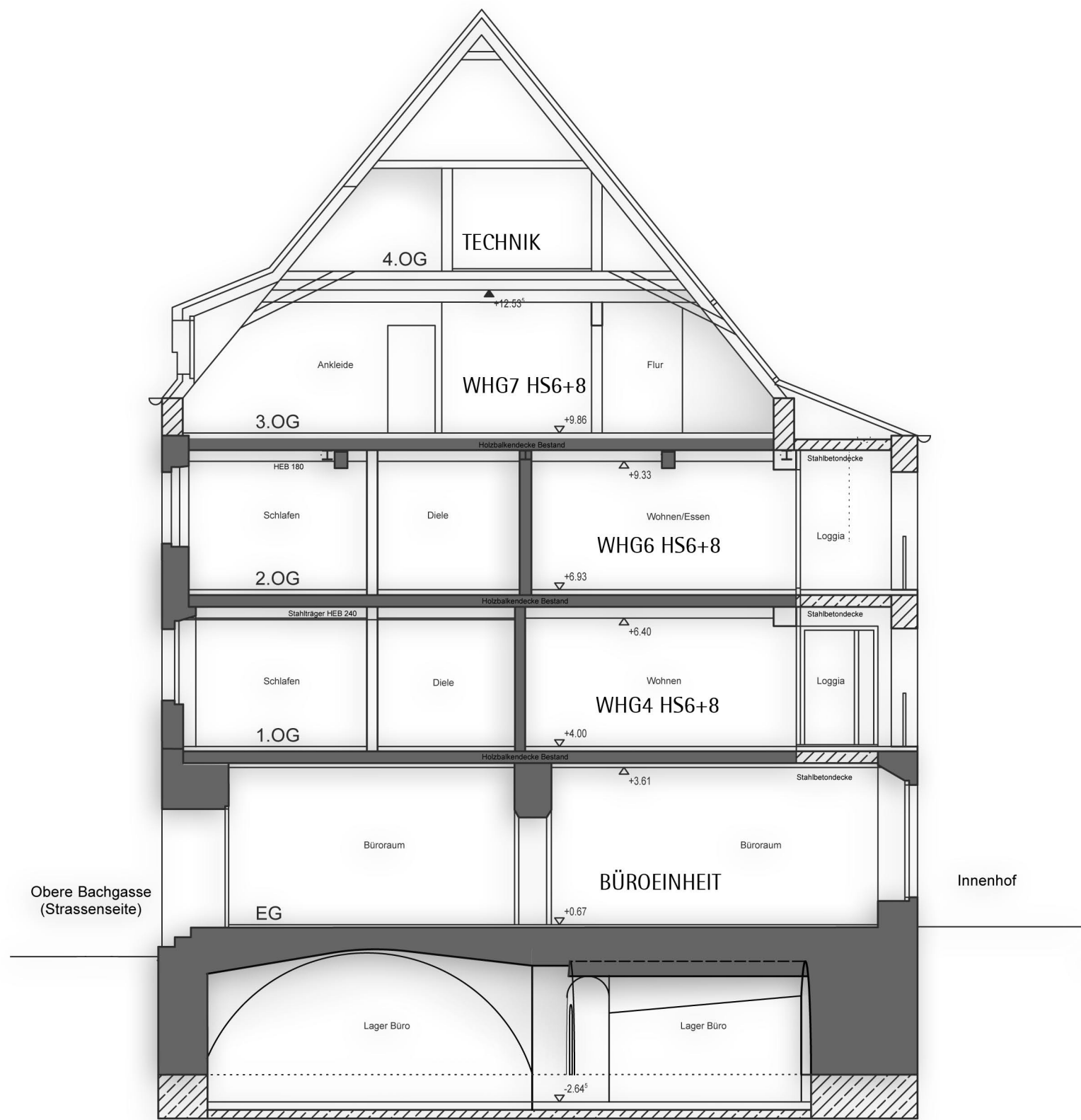
QUERSCHNITT HAUS 6 (DENKMAL) QS1
