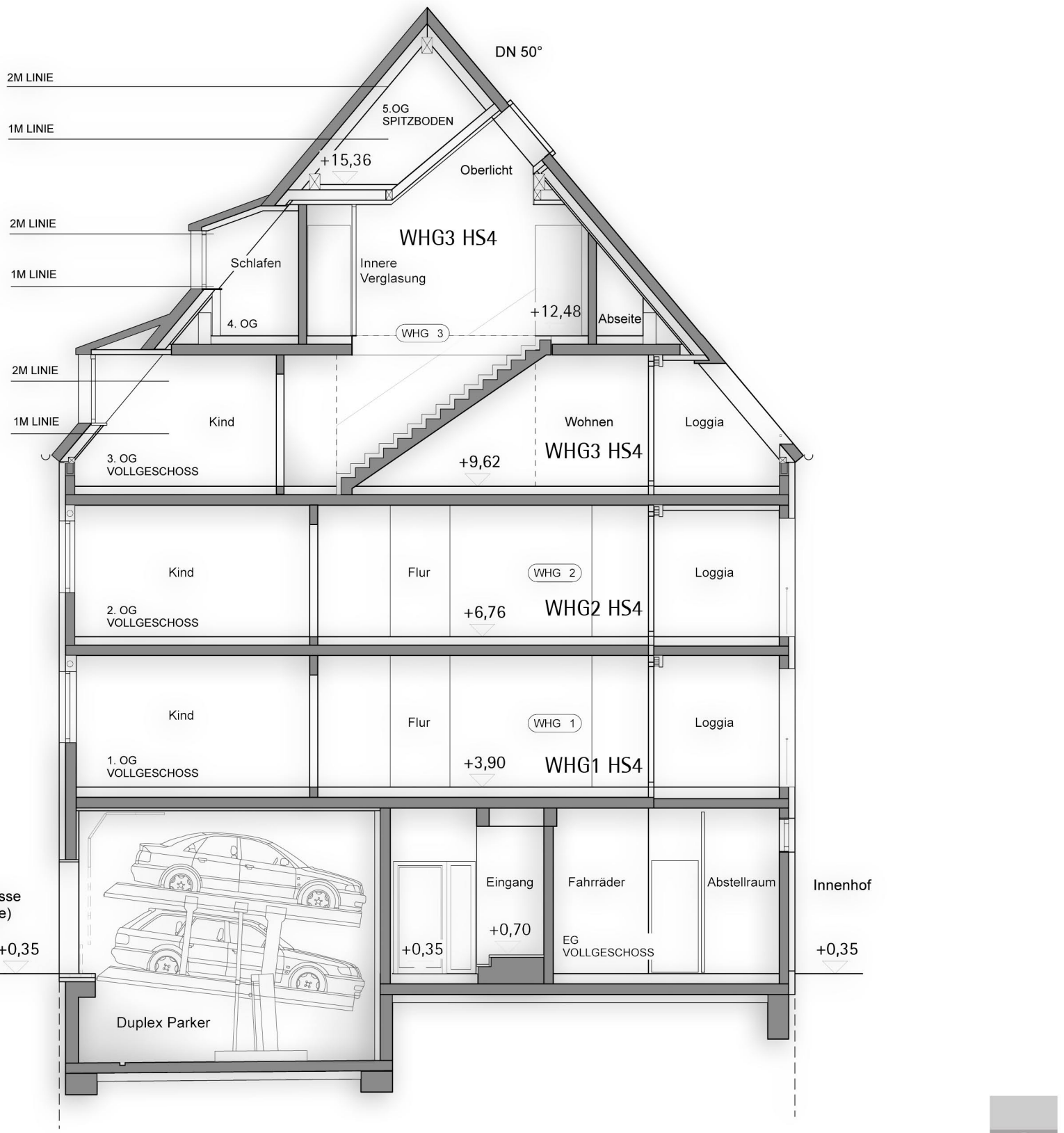
QUERSCHNITT HAUS 4 (NEUBAU) QS2
